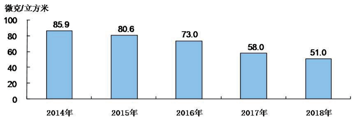
图10 2014-2018年细颗粒物（PM2.5）年均浓度
