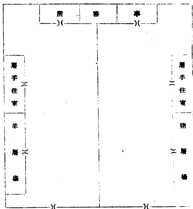
密雲縣政府修建石匣鎮屠宰場房增平面圖
